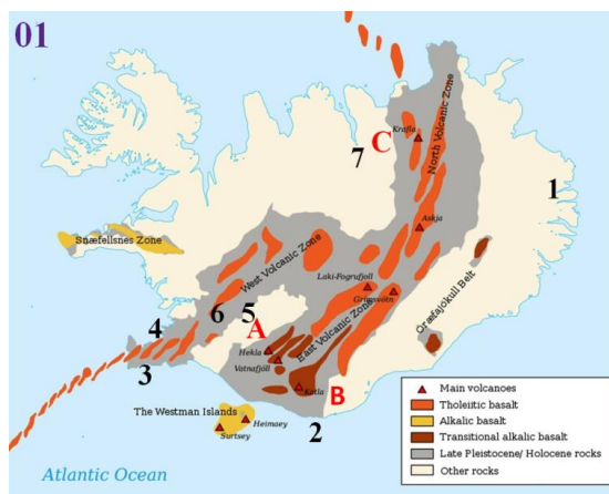
Fig. 01. Strefy wulkaniczne Islandii. Kolory żółty, pomarańczowy i brązowy – skały bazaltowe o różnych składach chemicznych; kolor szary – skały młodsze niż 2,5 mln lat. A – wulkan Hekla, B – wulkany Katla i Eyjafjallajökull, C – wulkan Krafla. 1 - Seyðisfjörður, 2 - Vík í Mýrdal, 3 - Grindavík i Błękitna Laguna, 4 - Reykjavík, 5 - Gullfoss, 6 - Gejzery Geysir i Strokkur, 7 - Akureyri.
